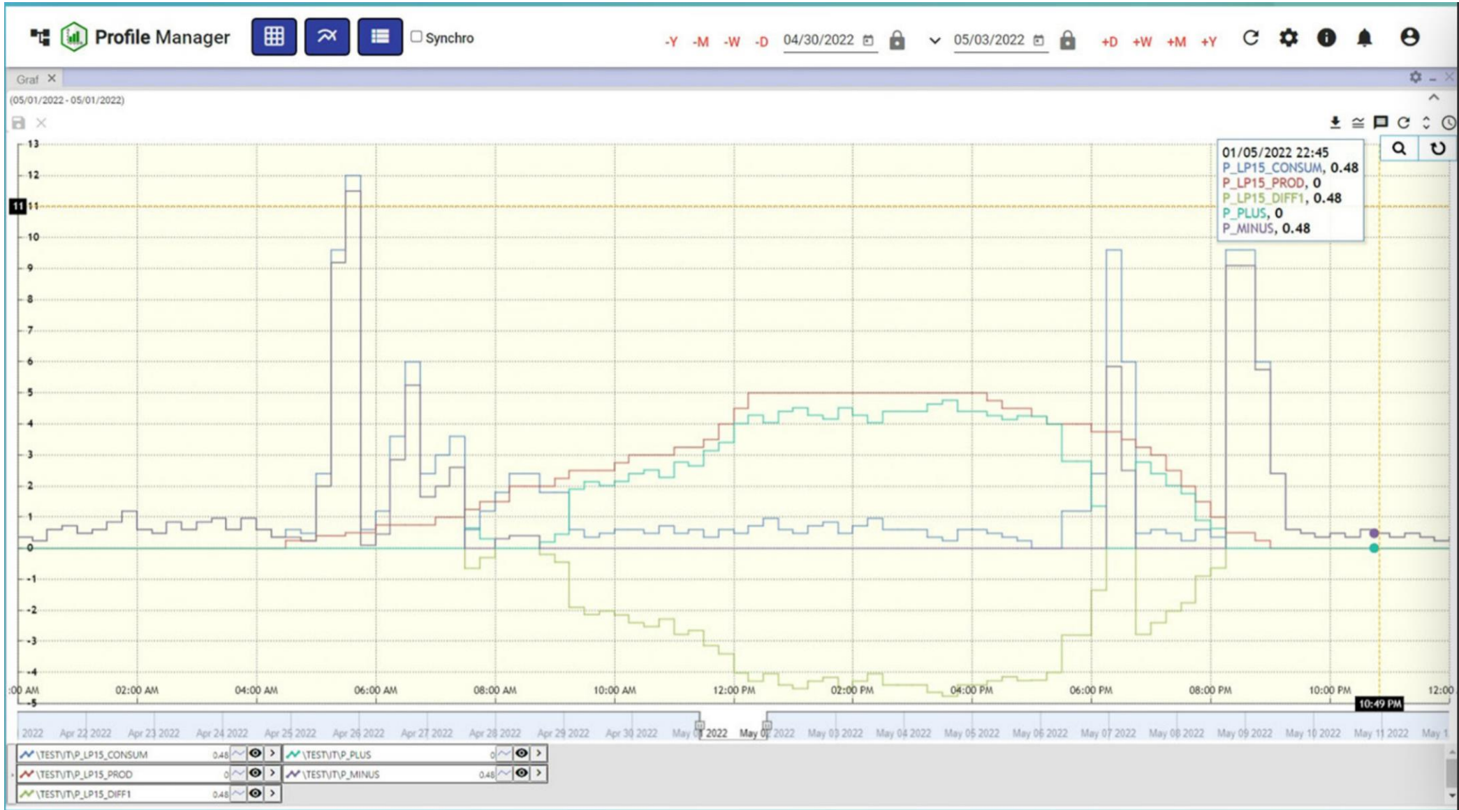
OZE a BESS prinášajú zmenu v dennom diagrame bilancie OOM (príklad domácnosti s FVE)
